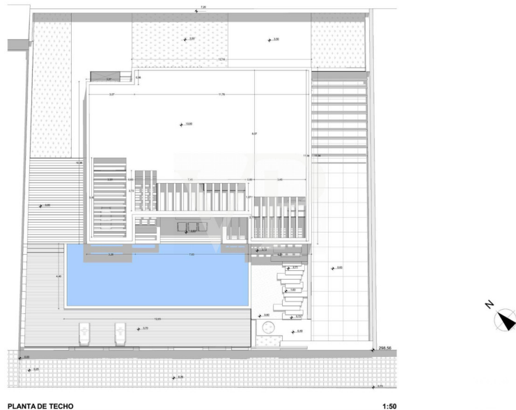
PLANTA DE TECHO 1:50
