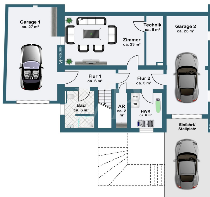
Kellergeschoss
