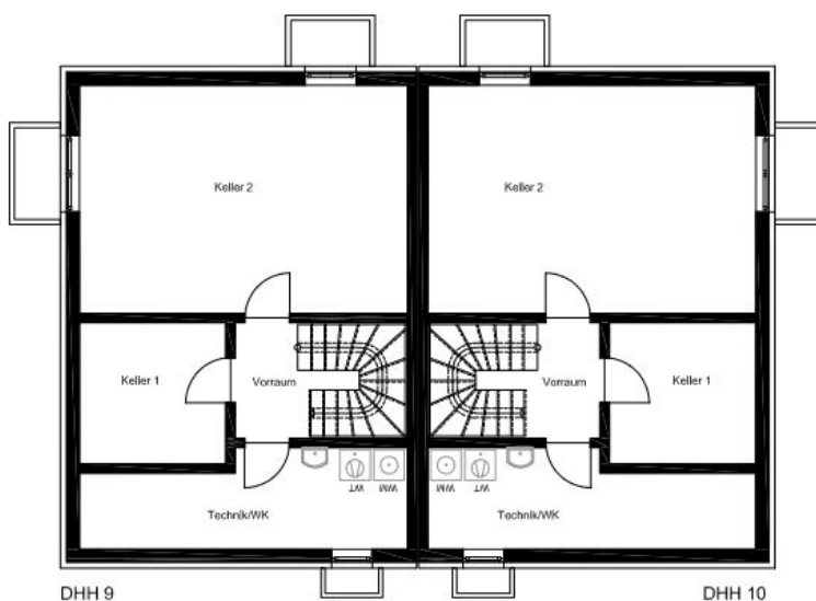
Grundriss UG
