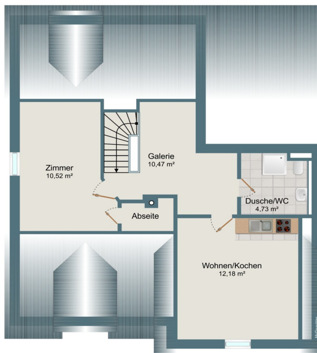
Dachgeschoss
