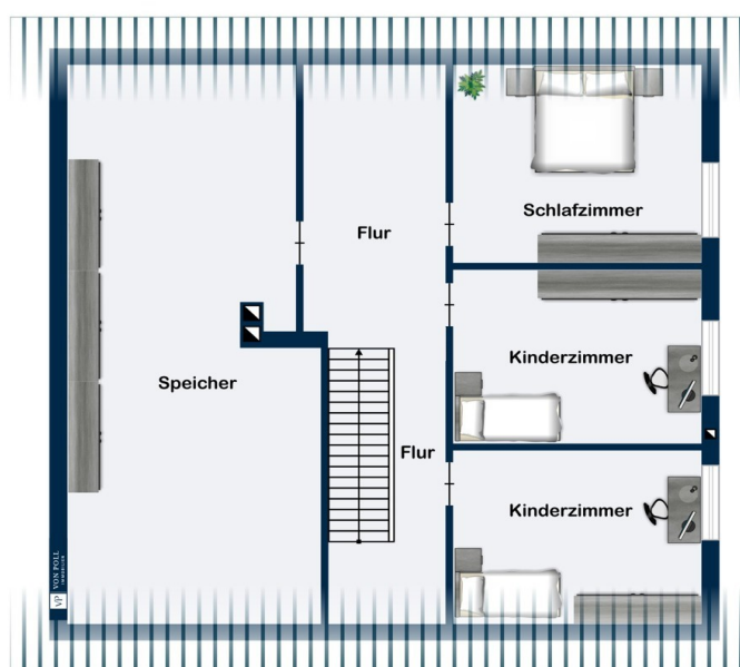
Dachgeschoss
