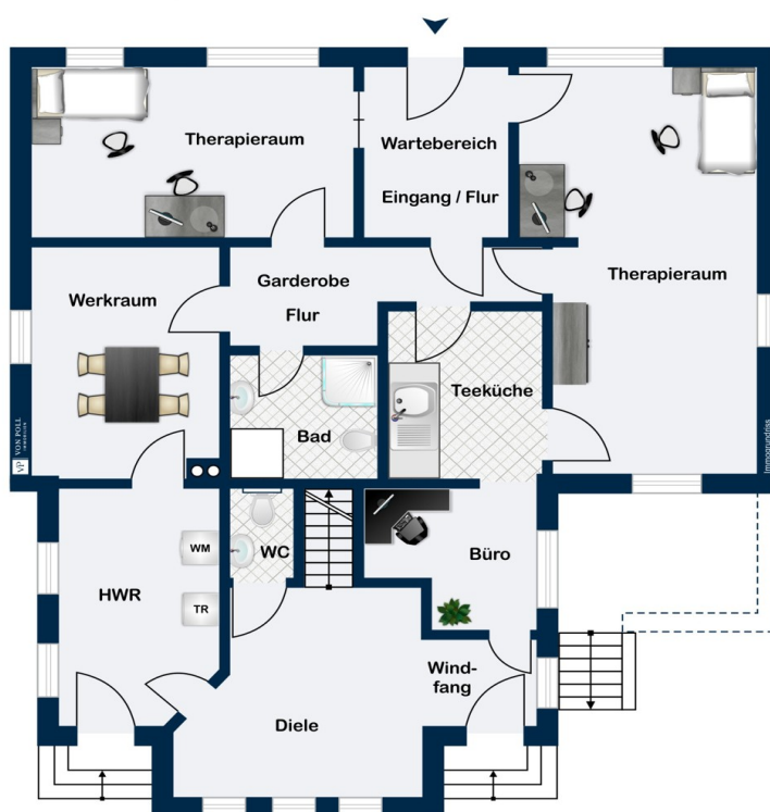
Erdgeschoss
