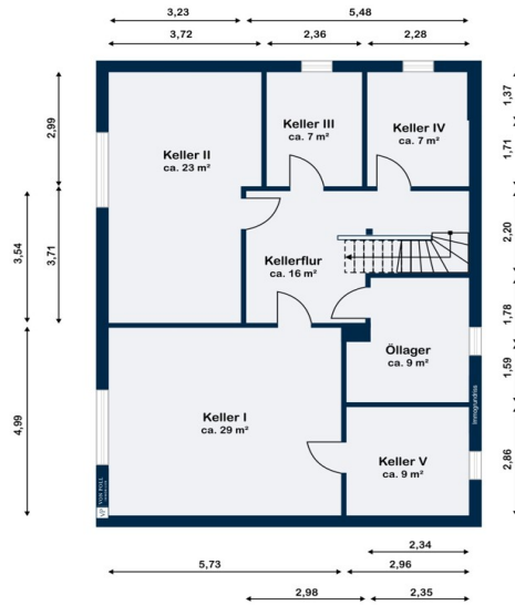
Kellergeschoss
