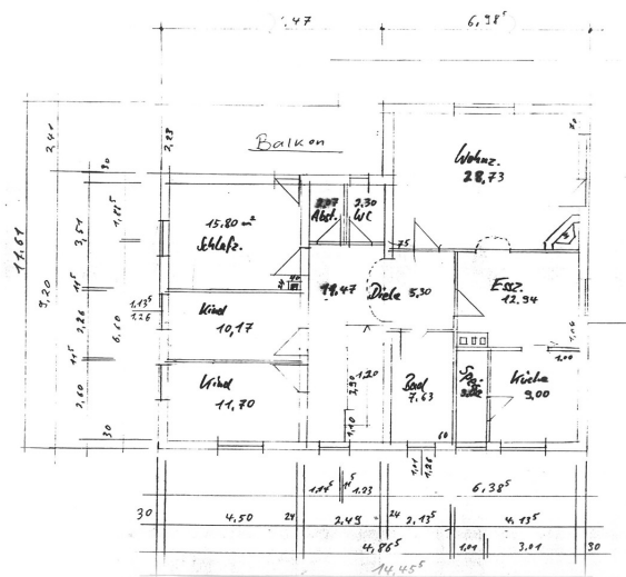
Grundriss Obergeschoss
