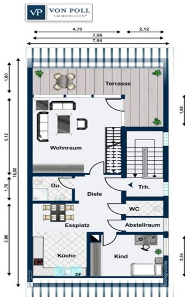
1.Dachgeschoss
